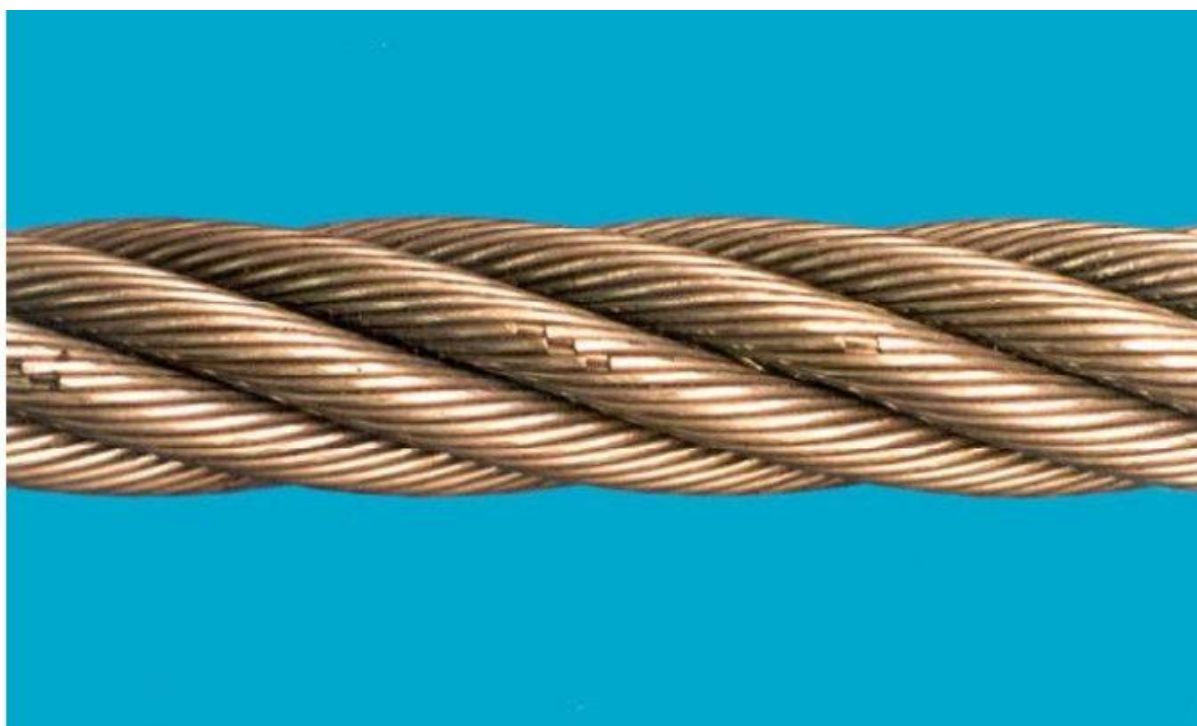
شکل ب ۱۳ - شکست سیم های تاج
