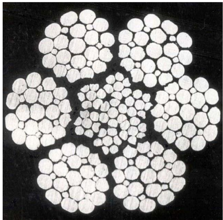
شکل ب ۱۹ - خوردگی درونی
