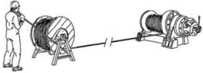
شکل ۴- مثالی از انتقال طناب سیمی از پایین عاسوره به پایین درام یا کشیدگی کنترل شده
