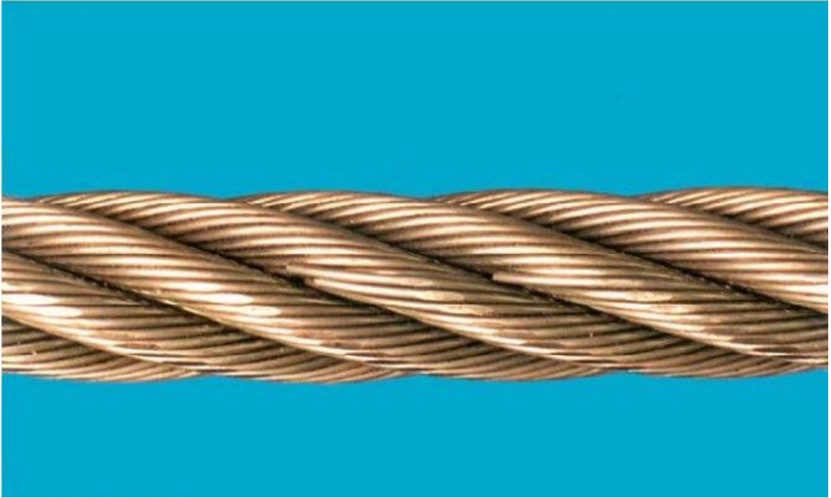
شکل ب ۱۴ - شکست سیم های شکاف
